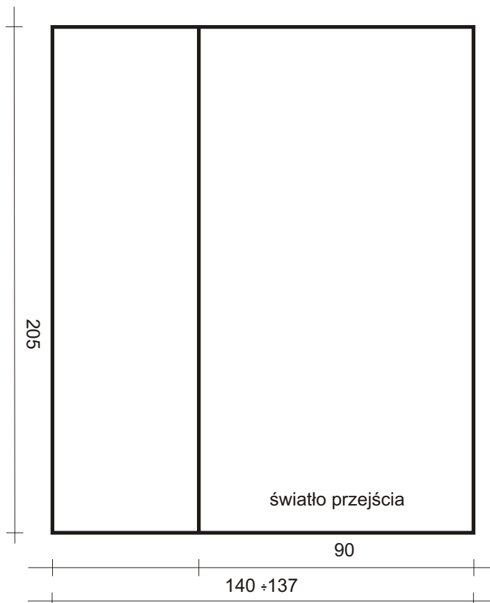
drzwi dwuskrzydłowe
