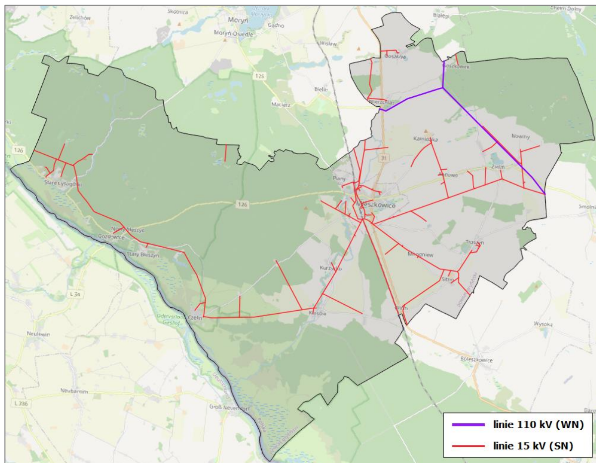
Rysunek 5. Przebieg napowietrznych linii elektroenergetycznych wysokiego (110 kV) i średniego (15 kV) napięcia na terenie gminy Mieszkowice
